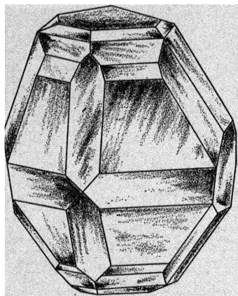
RHOMBIC
