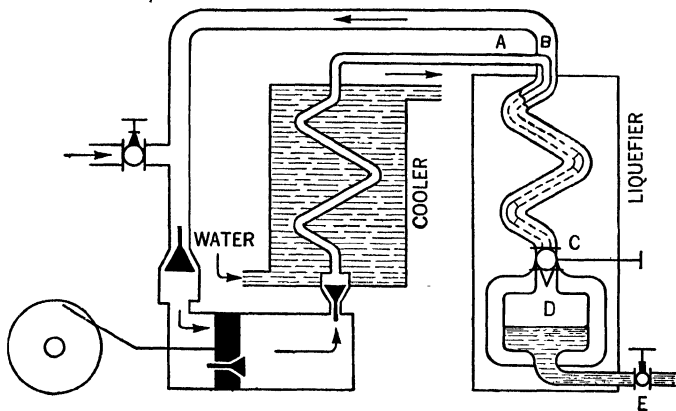
FIG. 47.—An air liquefier.
